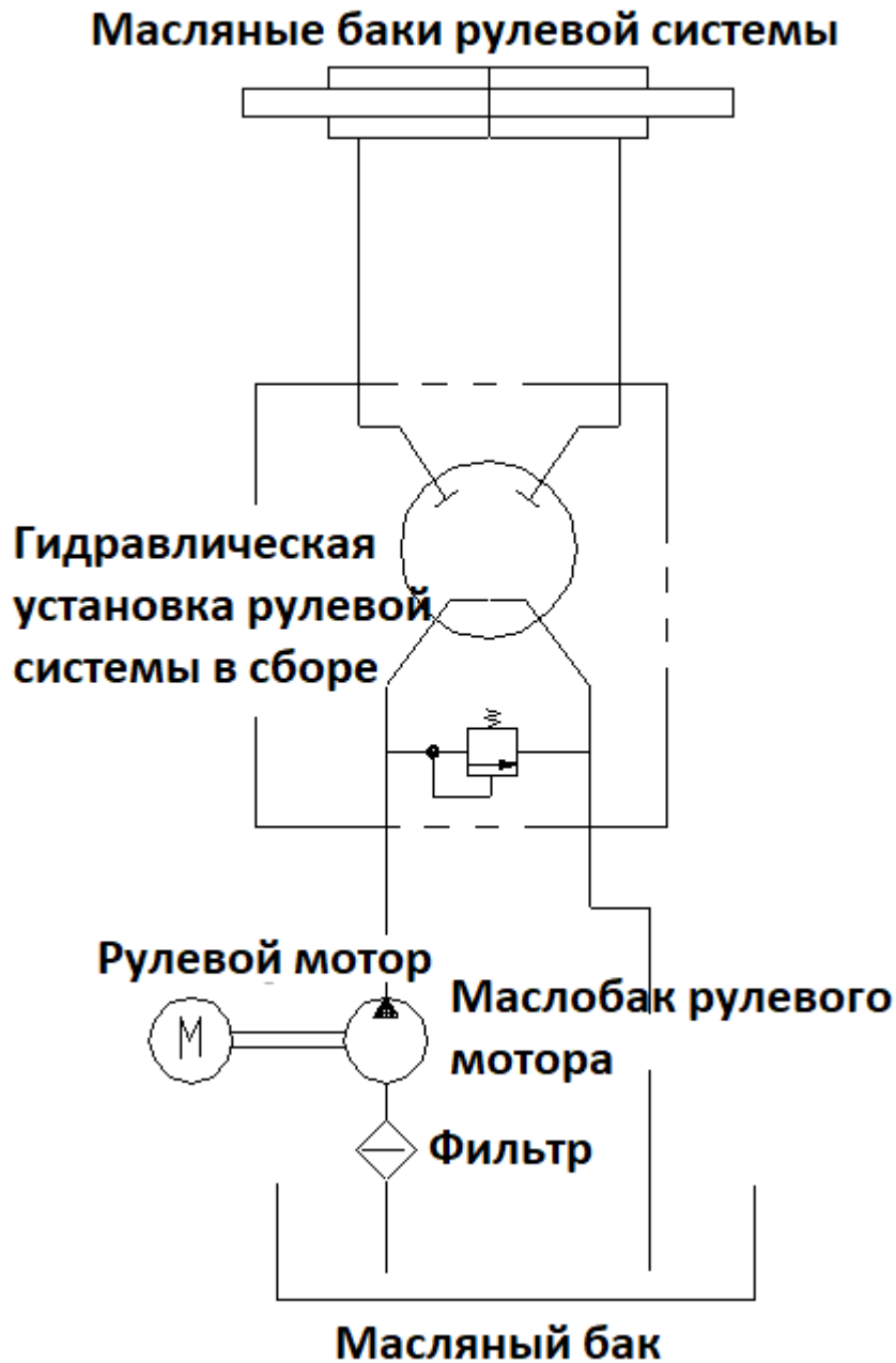
Рис. 12 – Гидравлическая схема
