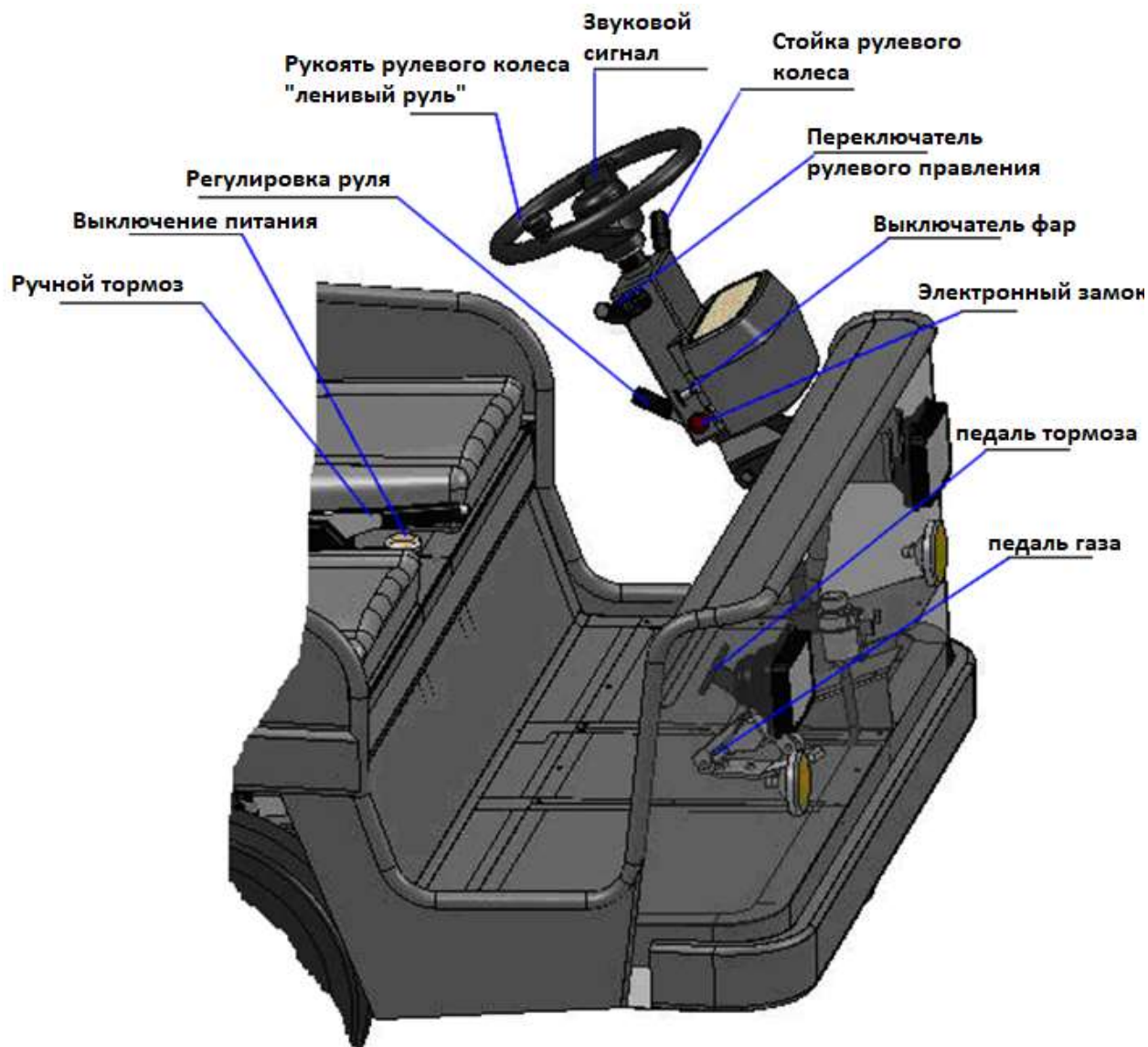
Рис. 1 – Элементы управления
