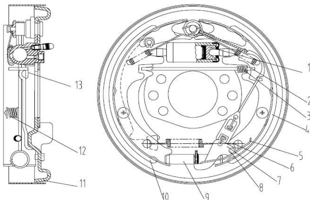
Рис. 6 – Барабанный тормоз
