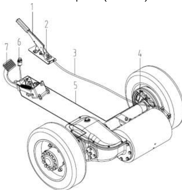
Рис. 9 – Тормозная система
