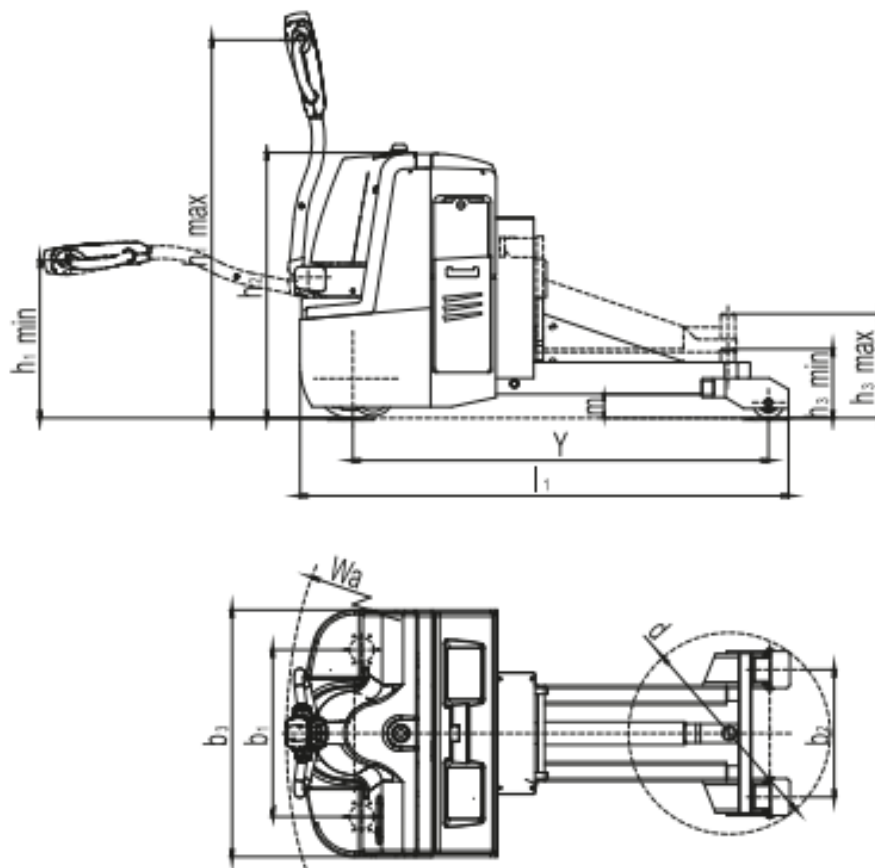
Рис. 1 – Общий вид и габаритные размеры
