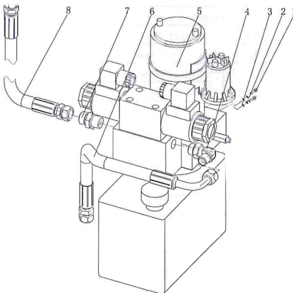
Взрыв схема 1
