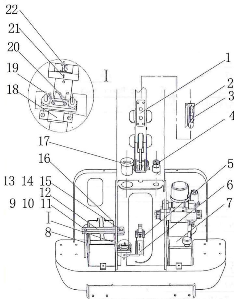
Взрыв схема 2
