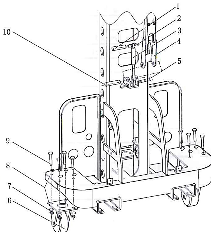
Взрыв схема 5
