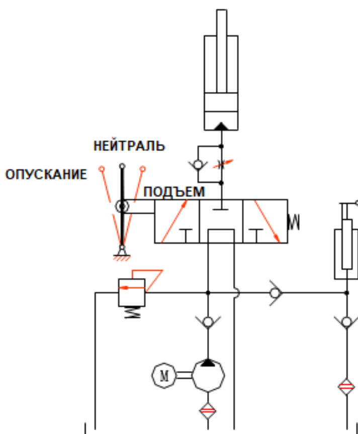
ГИДРАВЛИЧЕСКАЯ СХЕМА
