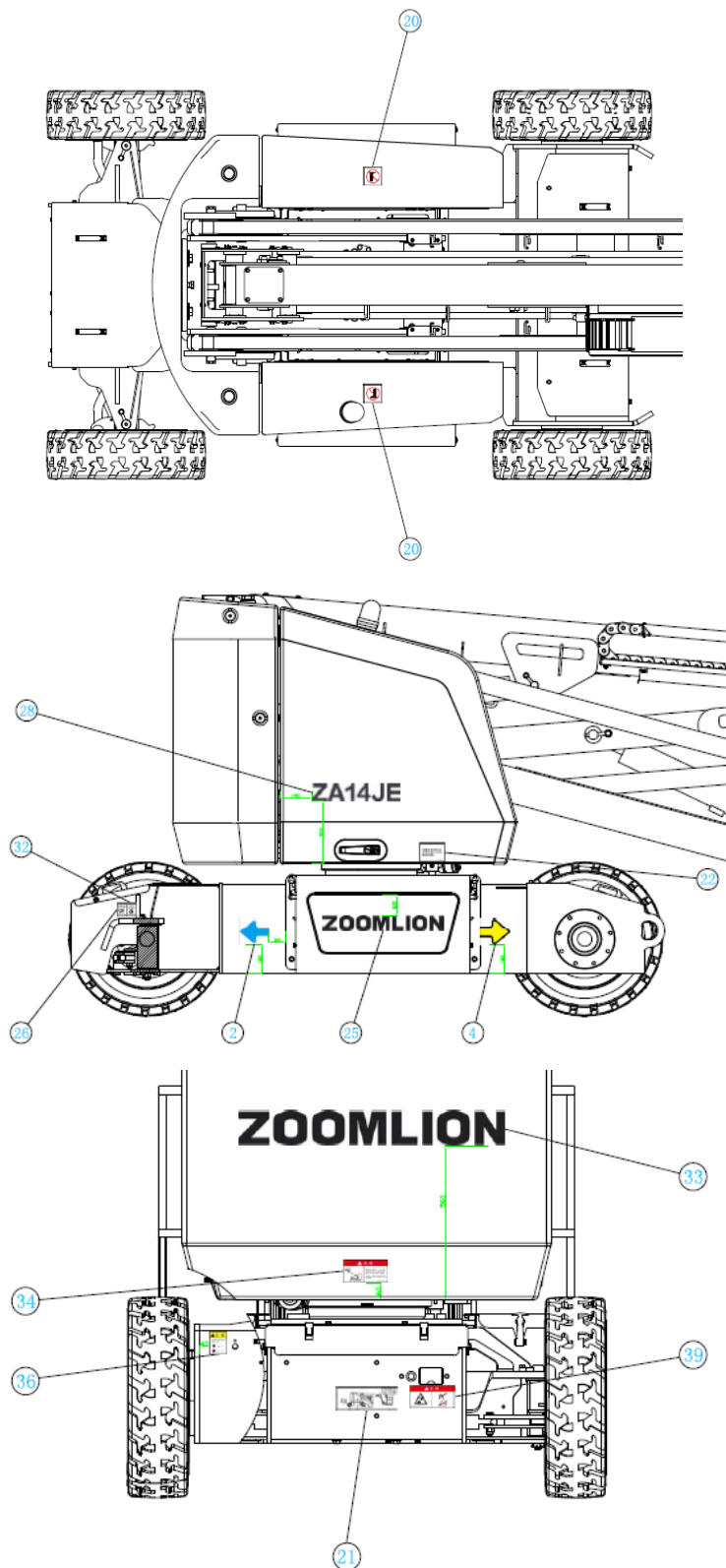
Рис. 3-1 Расположение маркировки
