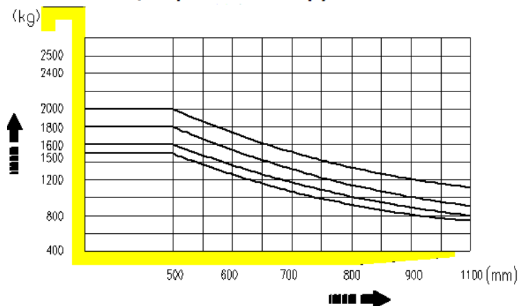
График зависимости грузоподъемности от центра тяжести груза на вилках
