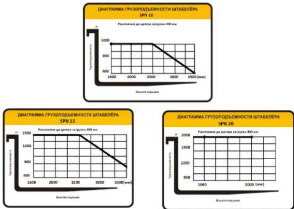
Рисунок. 4. Диаграмма грузоподъемности штабелера.
