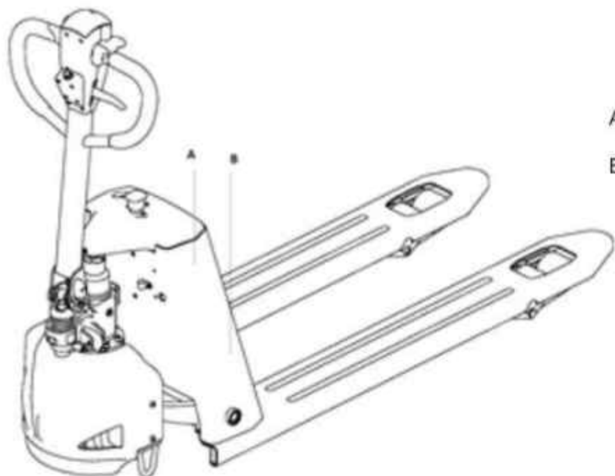
Рисунок.2. Предупреждающая маркировка.
