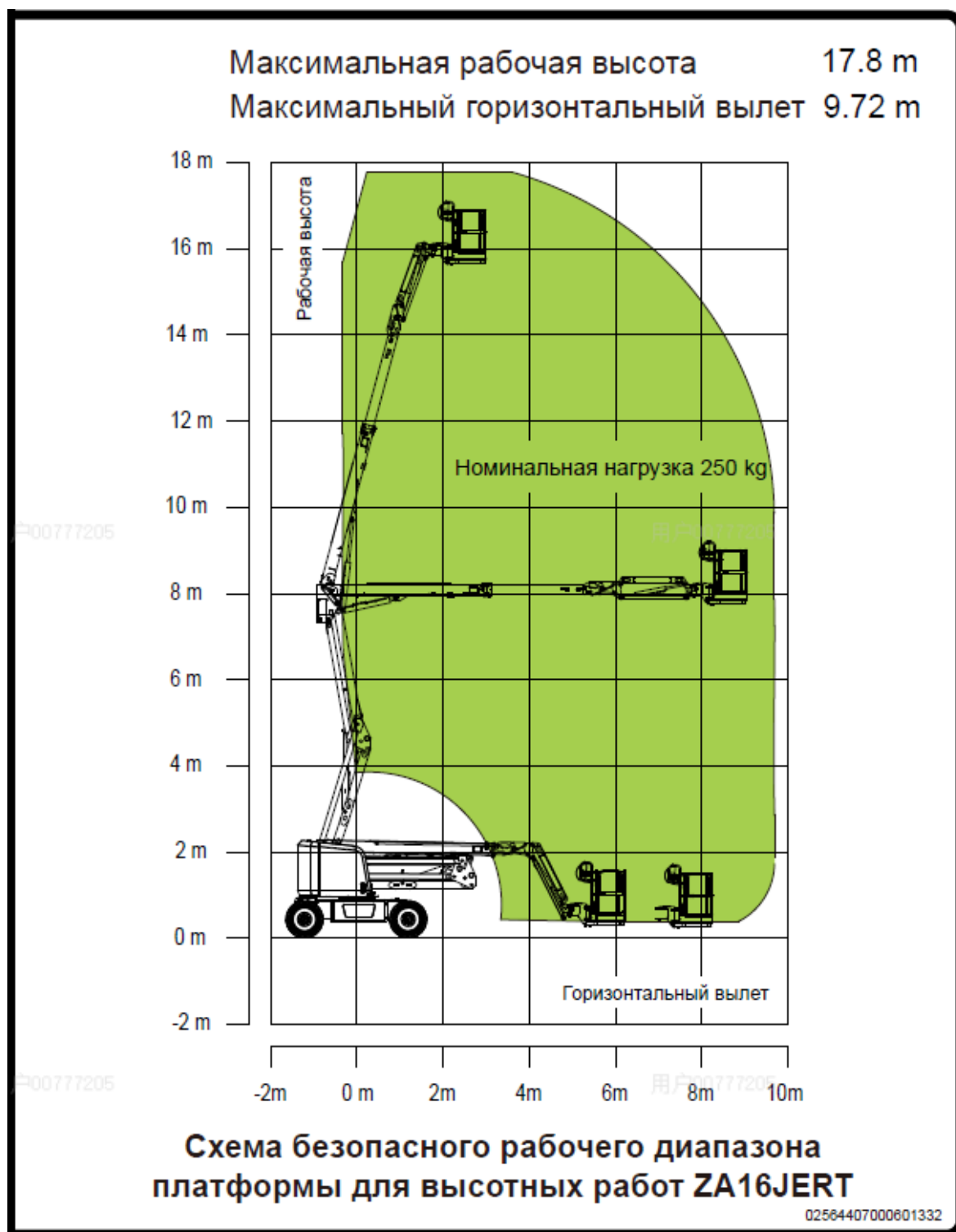
Рис. 7-1. Безопасный рабочий диапазон подъемника для высотных работ ZA16JERT-
