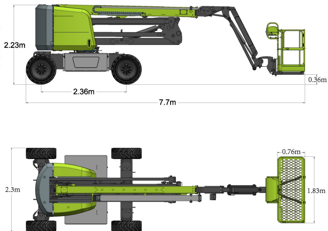
Рис. 7-2. Размеры в состоянии движения подъемника для высотных работ ZA16JERT
