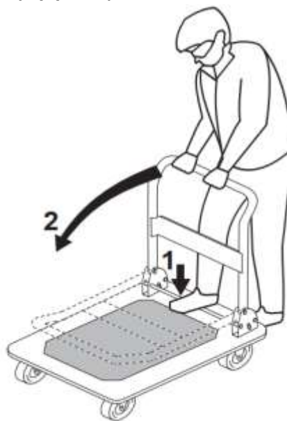
Рис. 1 – Складывание тележки
