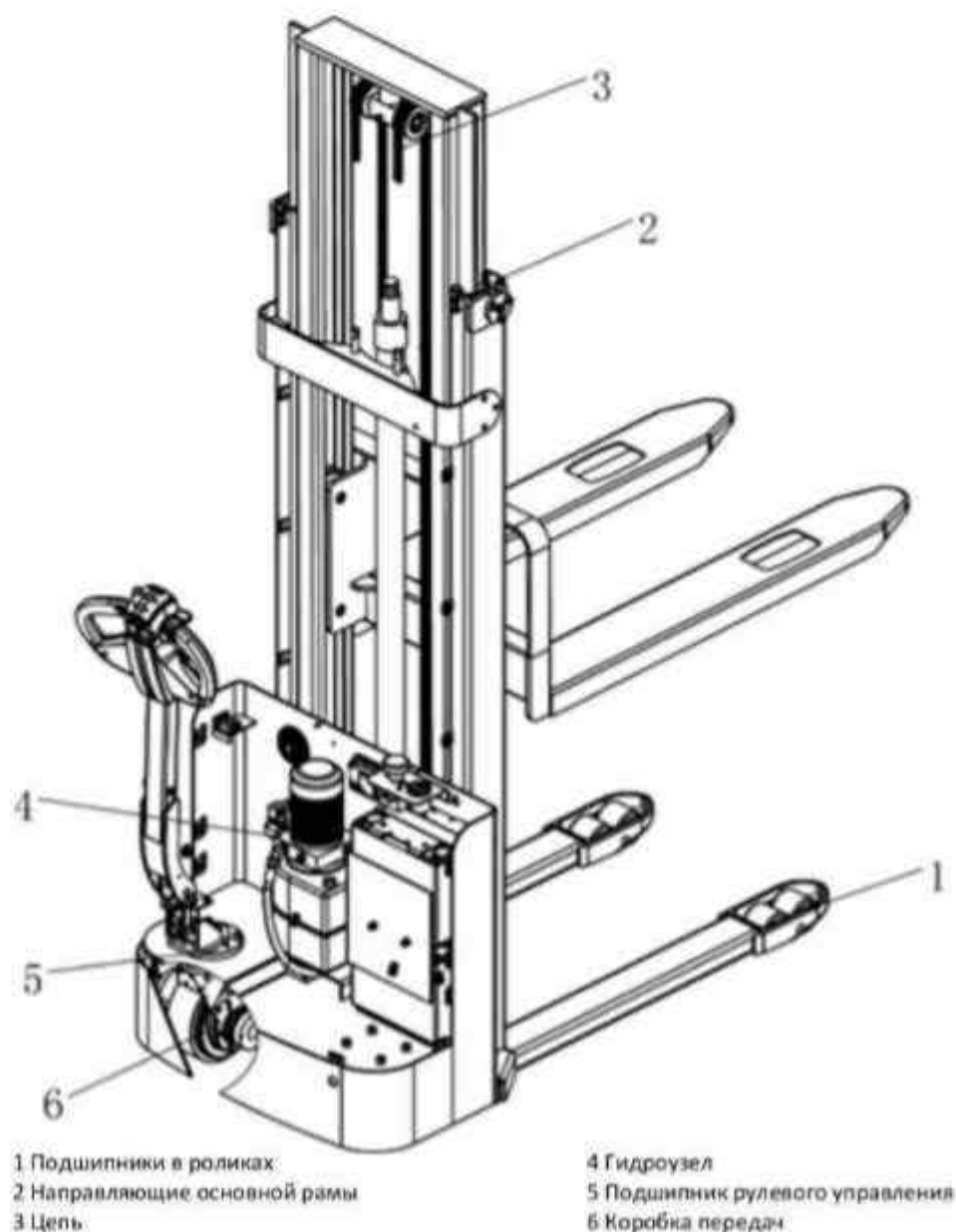
Рисунок 12. Основные точки смазки.
