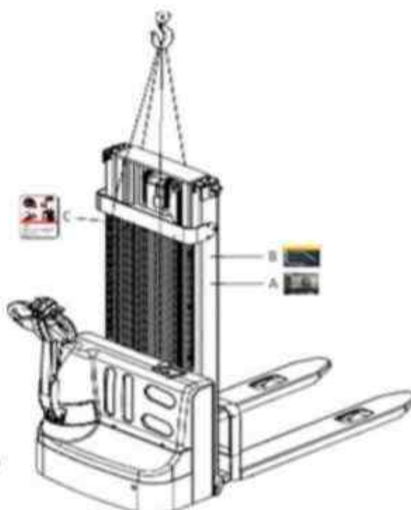
Рисунок 2. Предупреждающая маркировка.
