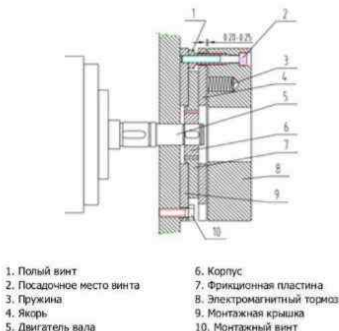
Рисунок 11. Регулировка зазора.
