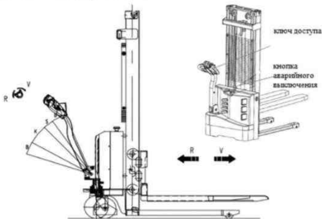
Рисунок 5. Органы управления.
