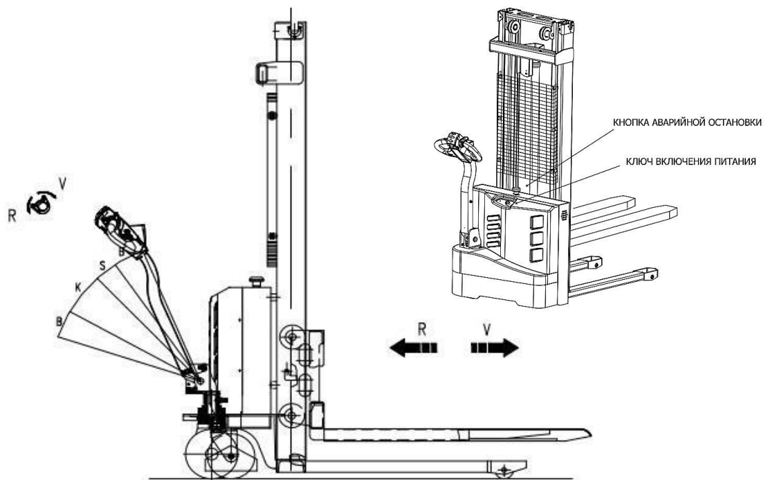
Рисунок 5. Органы управления.
