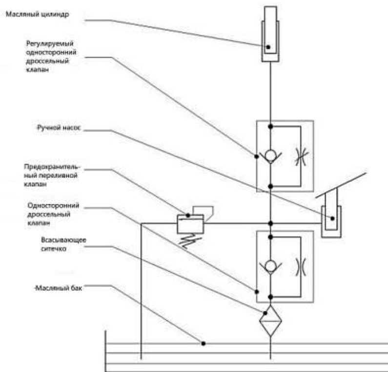
Рис.1 - Схема гидравлической системы
