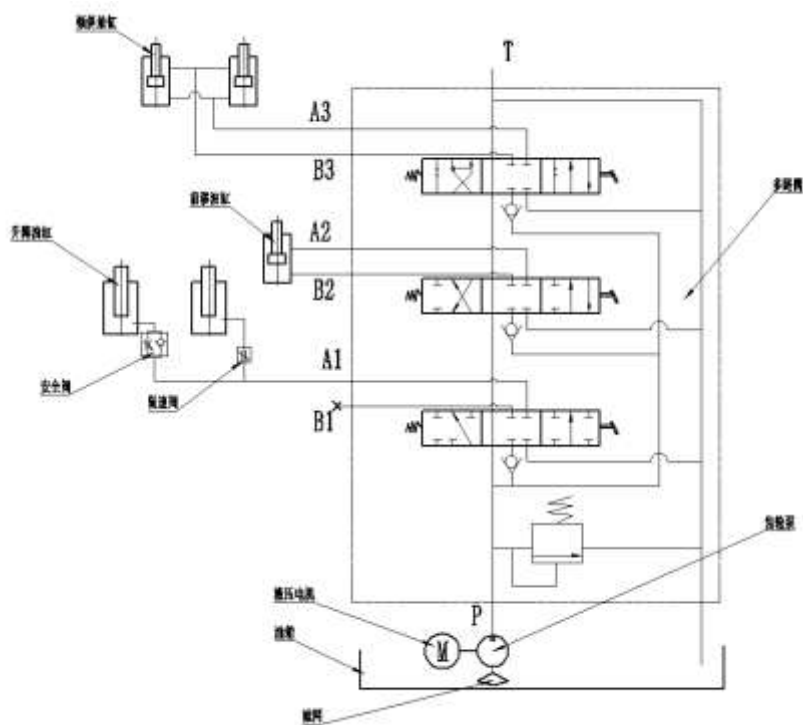
Рис. 4 Гидравлическая схема ричтрака CQD15T
