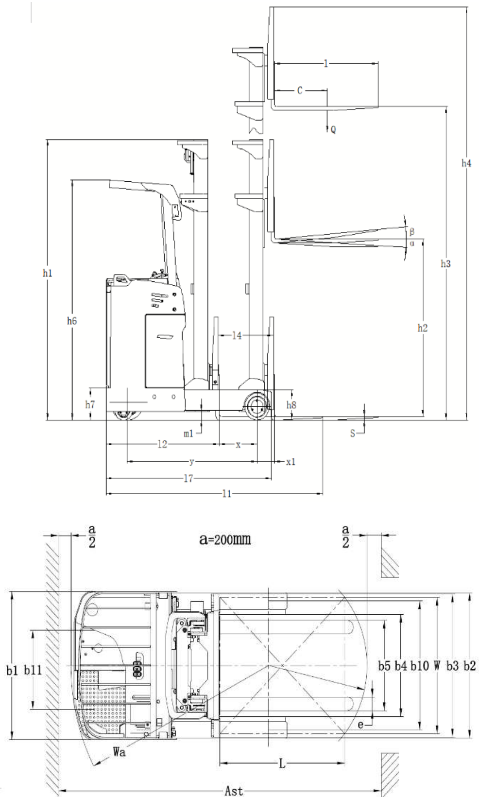
Рис. 1 Габаритный чертеж ричтрака CQD15T
