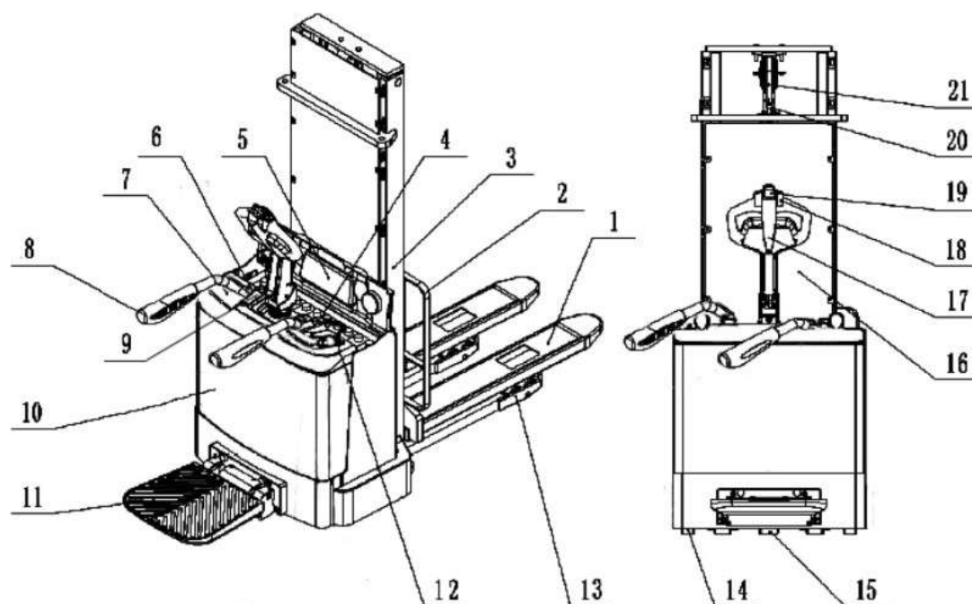
Рисунок. 1. Обзор основных компонентов.
