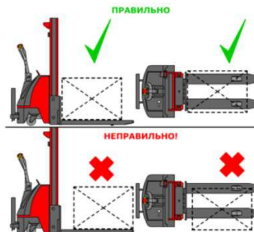
Рисунок 7. Схема расположения груза на вилках.
