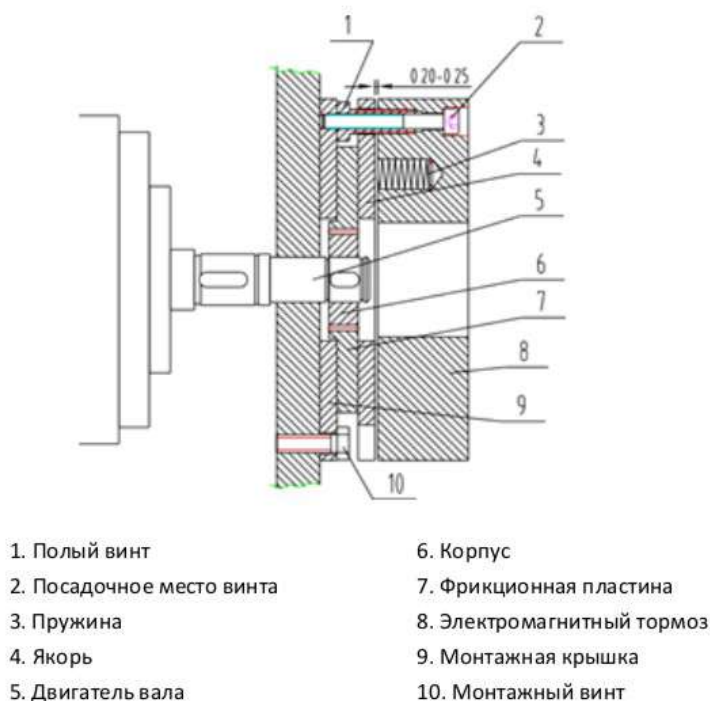
Рисунок 12. Тормозной механизм.
