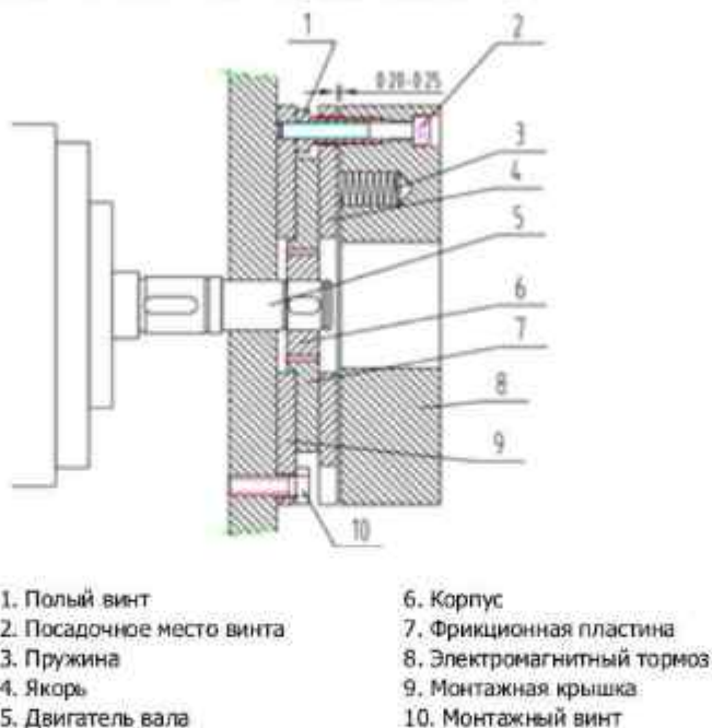
Рисунок 11. Регулировка зазора.
