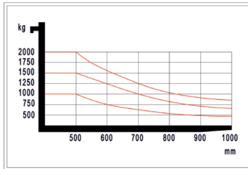
График грузоподъемности
