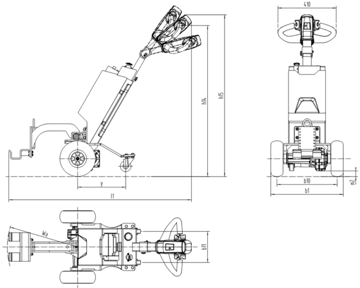
Рис. 1 – Общий вид и габаритные размеры
