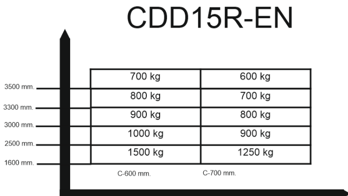
Рис. 2 и 3 – Кривые грузоподъемности
