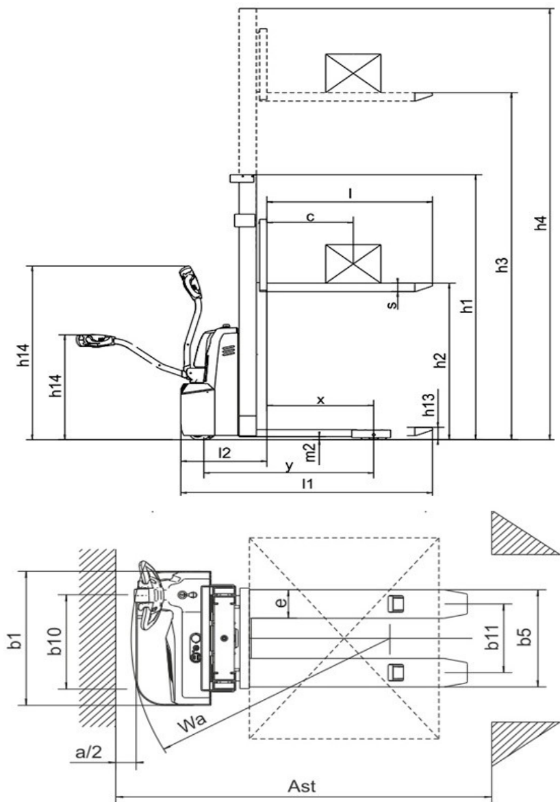
Рис.1 Габаритные размеры
