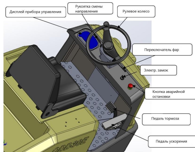
Рис. 2 – Элементы управления
