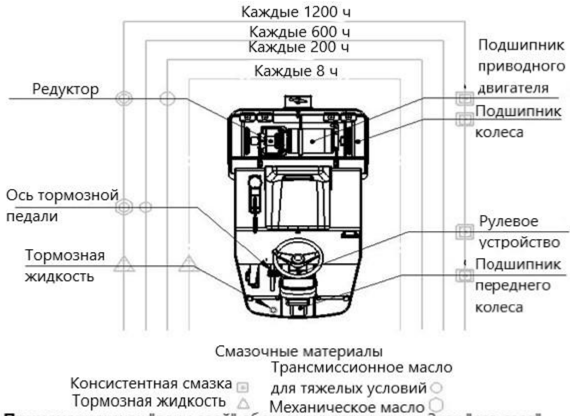
Рис. 5 – Схема смазки
