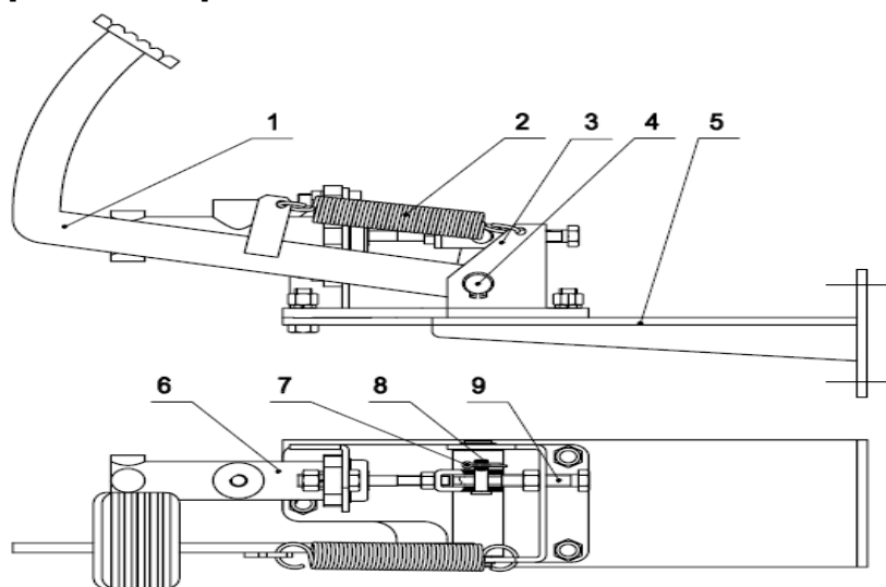
Рис. 12 – Ножной тормоз
