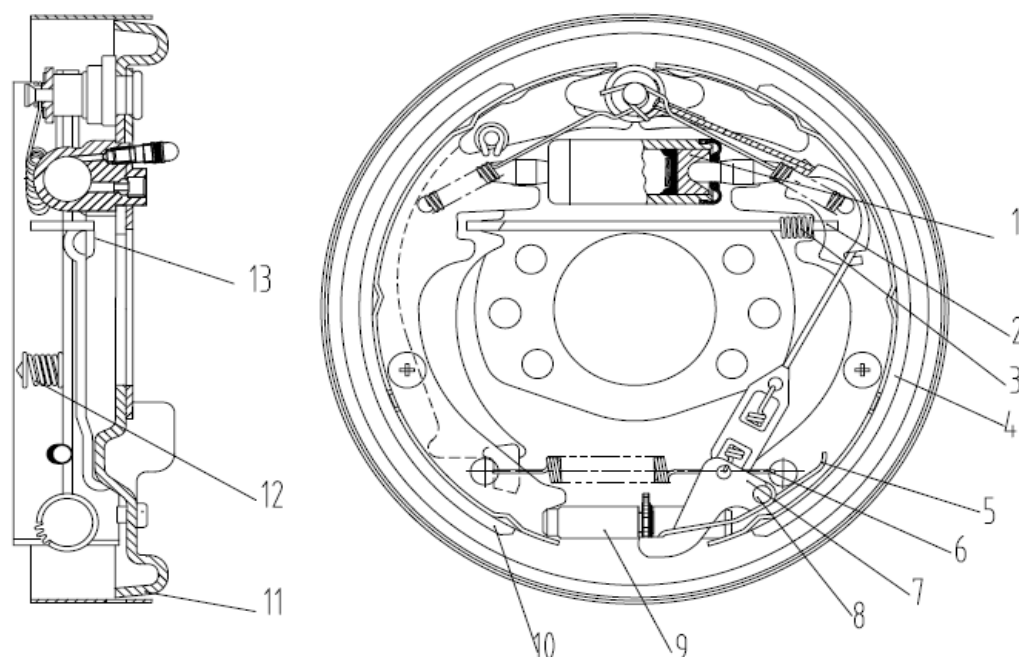
Рис. 7 – Барабанный тормоз
