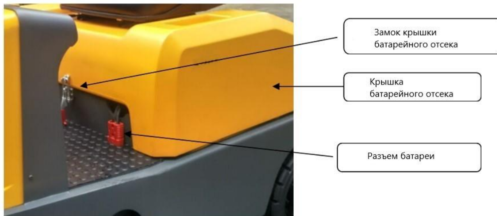
Рис.4 – Батарейный отсек
