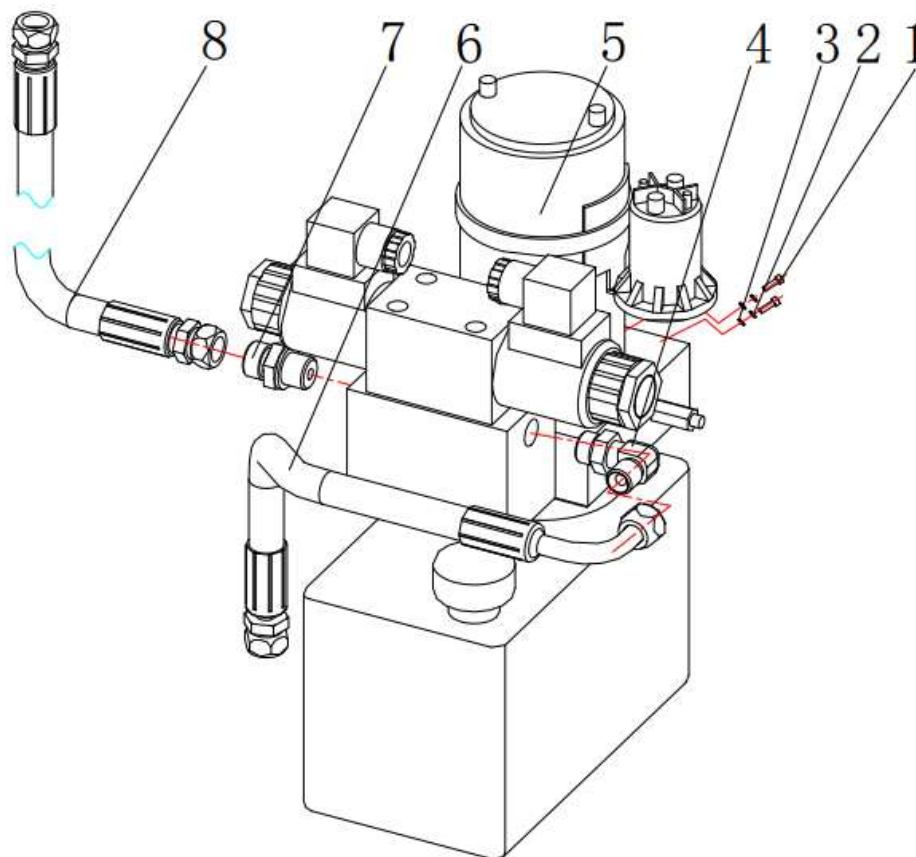
Взрыв схема 1
