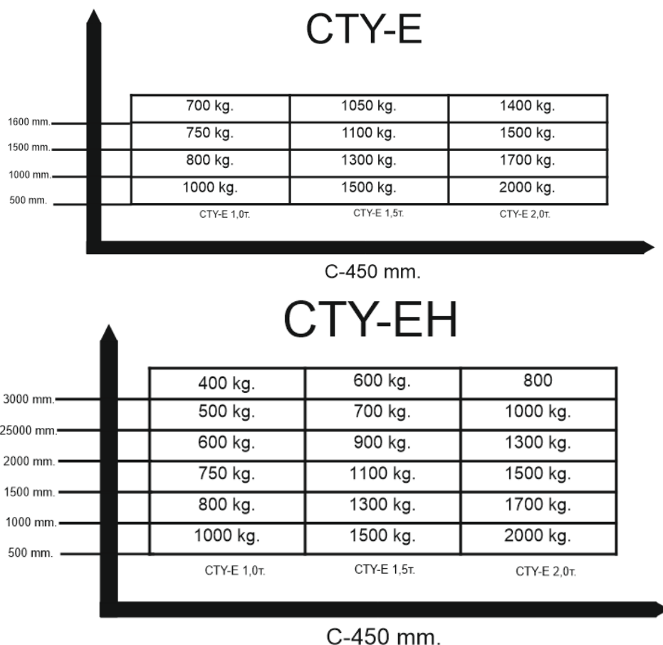
Рис. 2 – Кривые грузоподъемности
