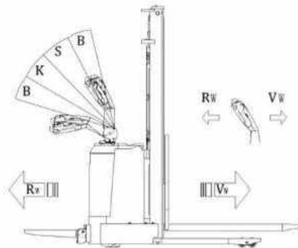
Рисунок 6 Положение румпеля управления.
