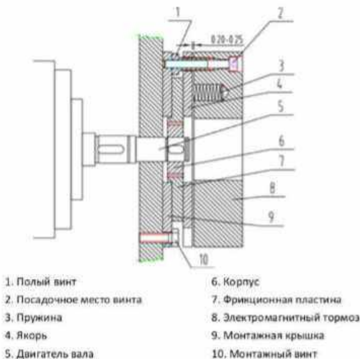
Рисунок 12. Тормозной механизм.
