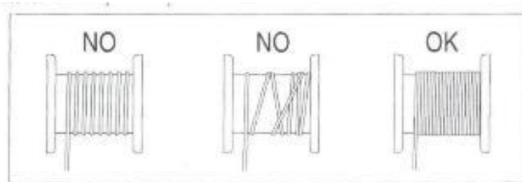
Рис.9 - Намотка троса на барабан
