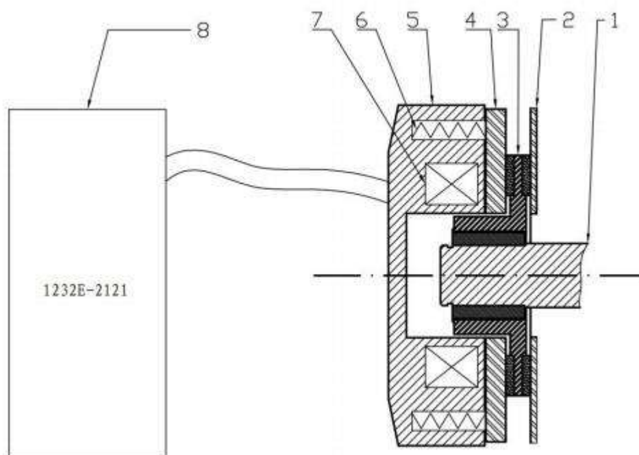
Рис. 9 – Тормозная система
