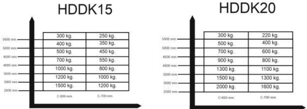
Рис. 2 – Кривые грузоподъемности
