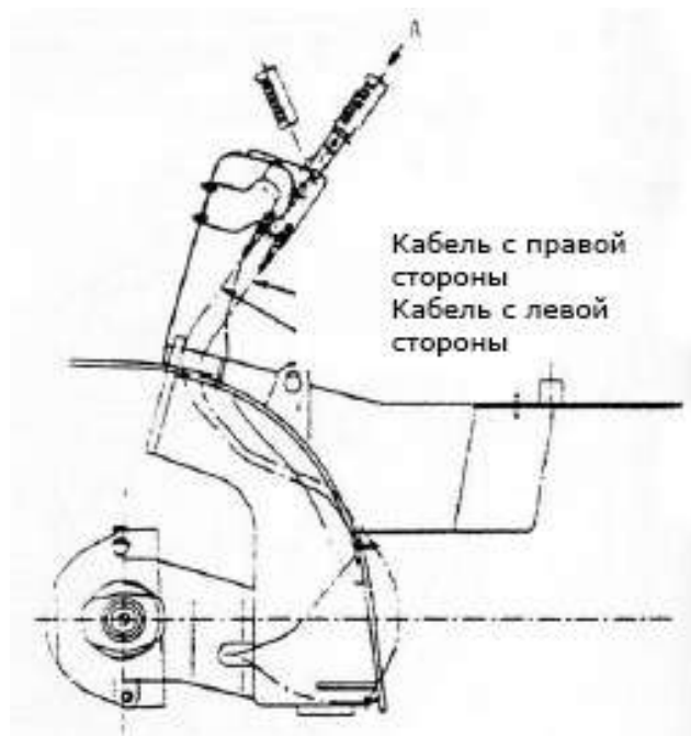
Рис.3-11 Ручка стояночного тормоза
