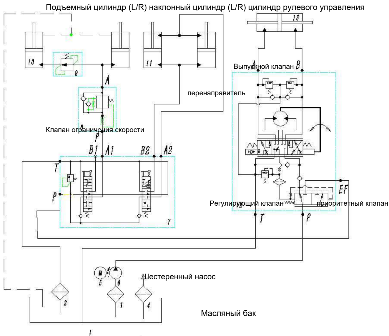
Рис. 3-37 гидравлическая система
