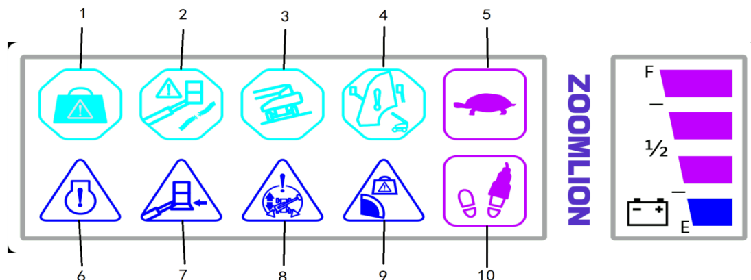
Рис. 2-10 Панель индикаторов платформы
