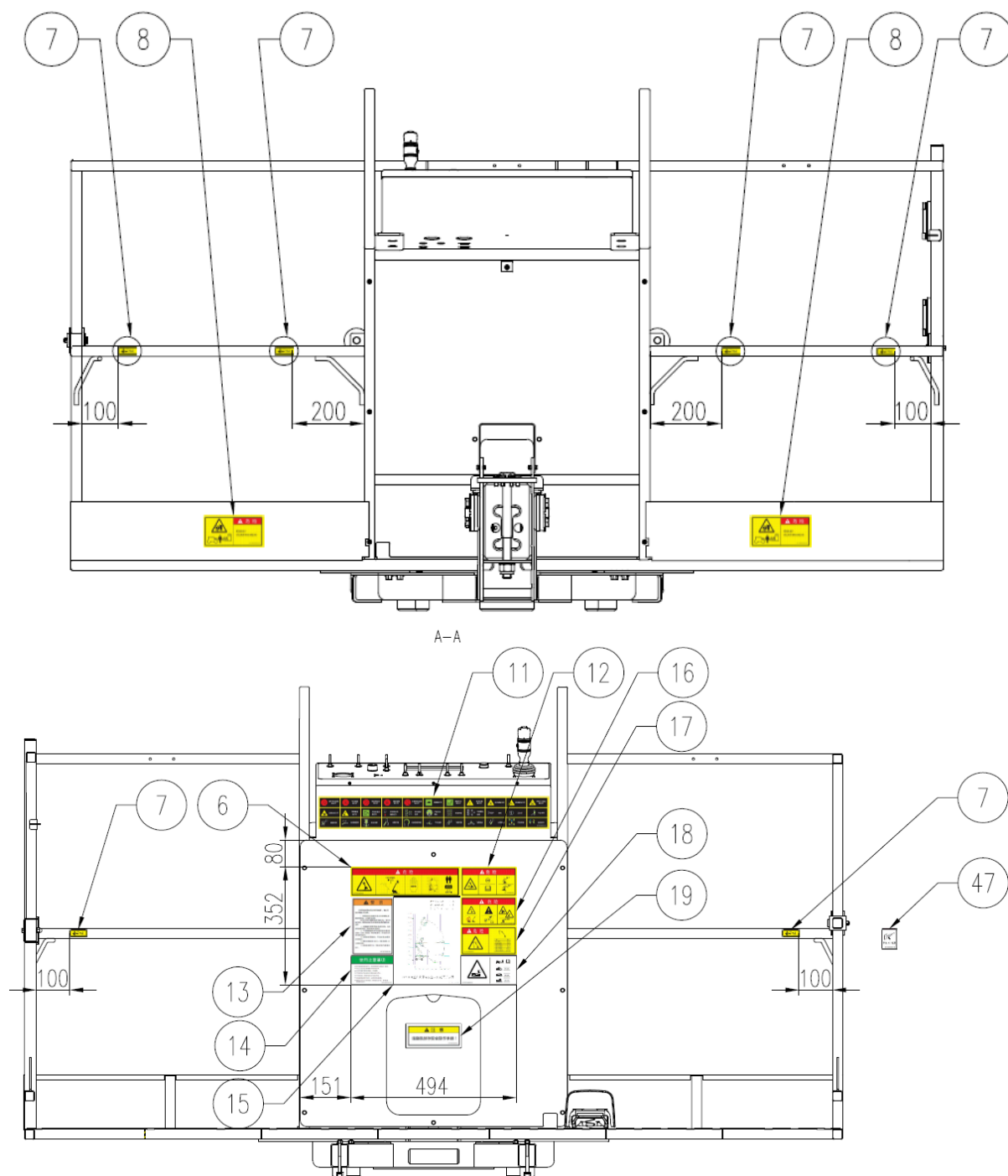
Рис. 3-1 Расположение маркировки (продолжение)
