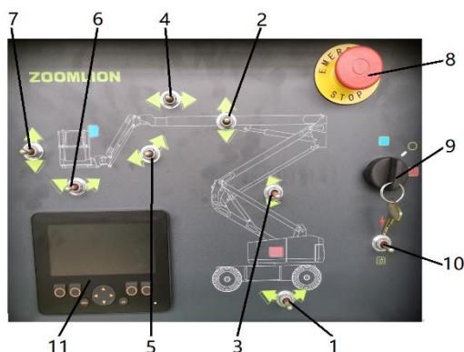
Рис. 2-2 Наземная панель управления
