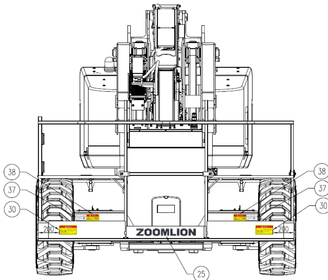
Рис. 3-1 Расположение маркировки (продолжение)
