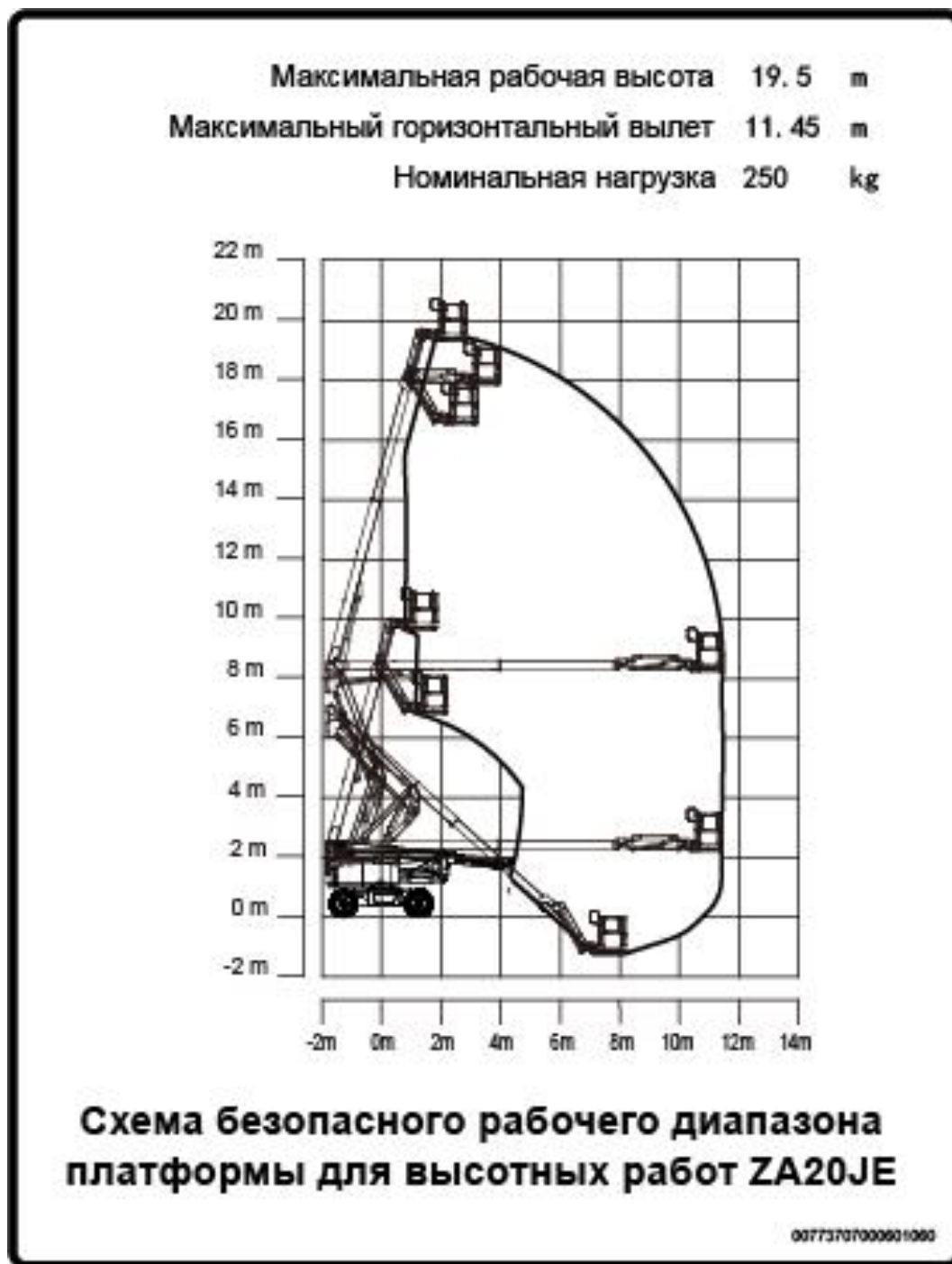
Рис. 7-1. Безопасный рабочий диапазон подъемника для высотных работ ZA20JE
