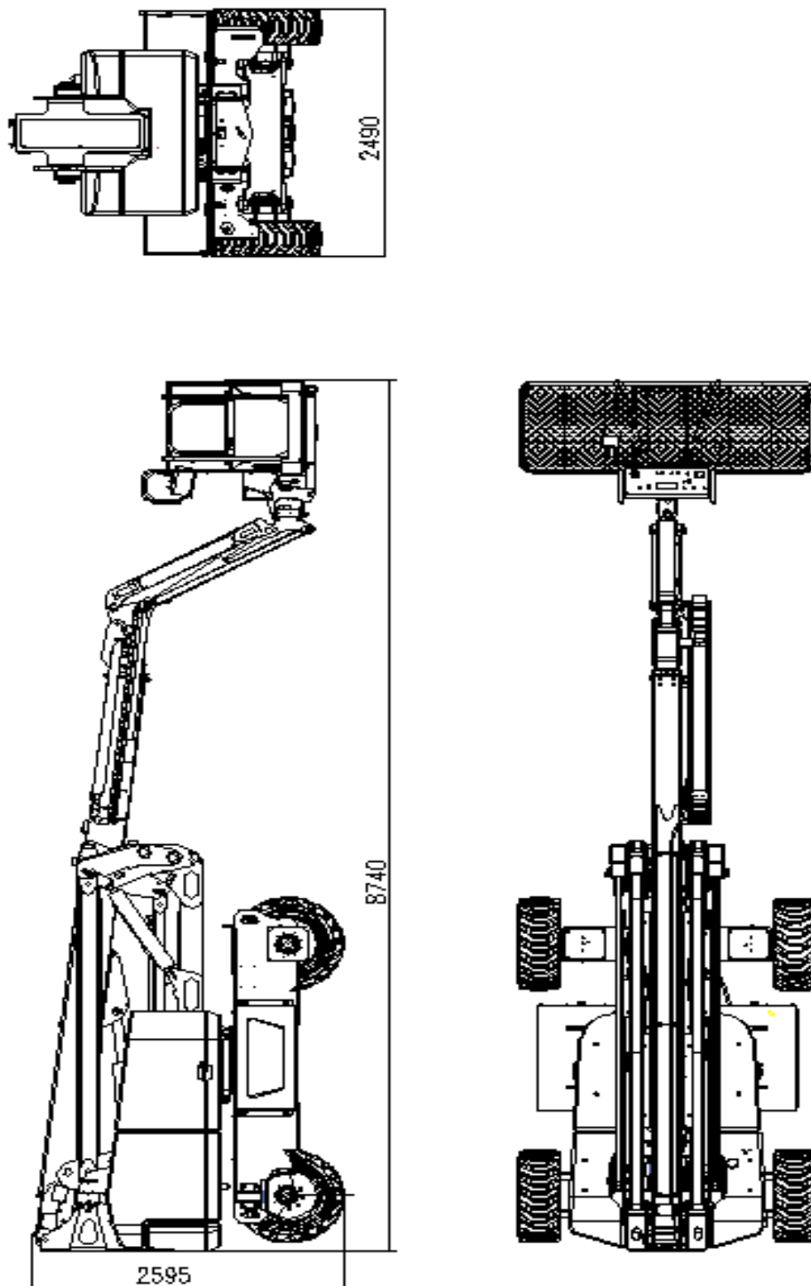
Рис. 7-2. Размеры в состоянии движения подъемника для высотных работ
