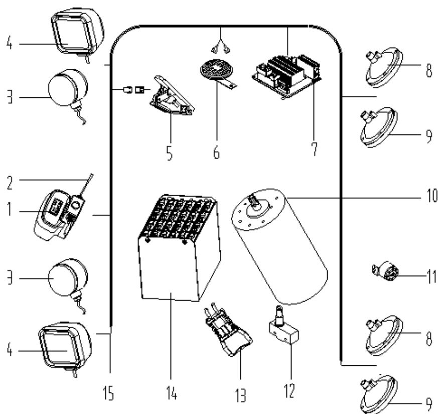
QDD20/30/50/60 Схема электрической системы
